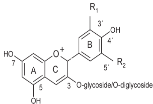
شکل ۴- ساختار شیمیایی آنتوسیانین‌های یافت شده در میوه‌های
