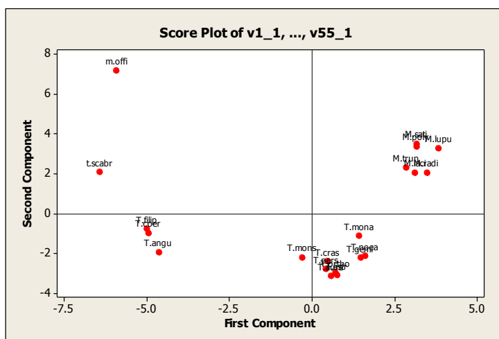
شکل ۲- نمودار حاصل از تجزیه به مؤلفه‌های اصلی (PCA) براساس صفات ریختی کمی و کیفی
